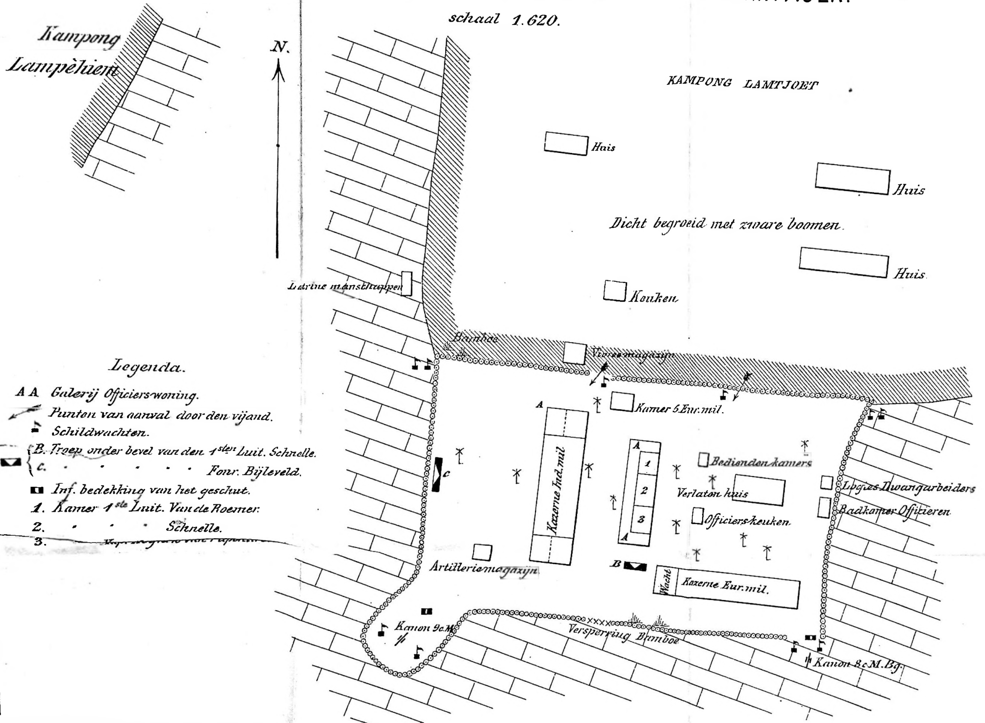
FIG. 1. SCHETS VAN HET VERSTERKT KAMPMENT TE LAMPAGER. schaal 1:620.
